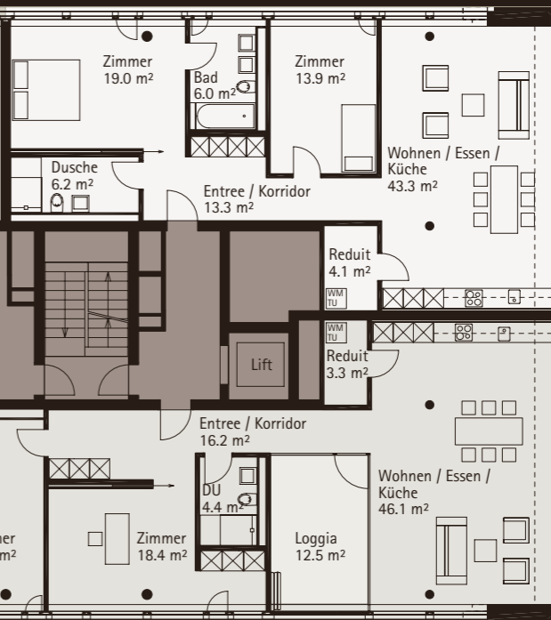
WOHNUNG 02.1101, 3 1/2-ZIMMER NGF: 116.2 m 2 , Loggia: 12.5 m 2
