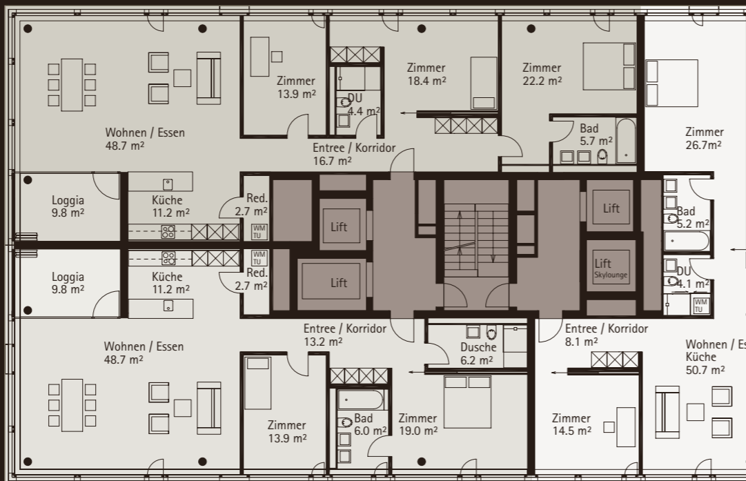
WOHNUNG 01.1002, 3 1/2-ZIMMER NGF: 121.0 m 2 , Loggia: 9.8 m 2
