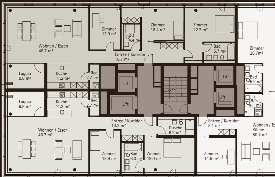
WOHNUNG 01.1102, 3 1/2-ZIMMER NGF: 121.0 m 2 , Loggia: 9.8 m 2
