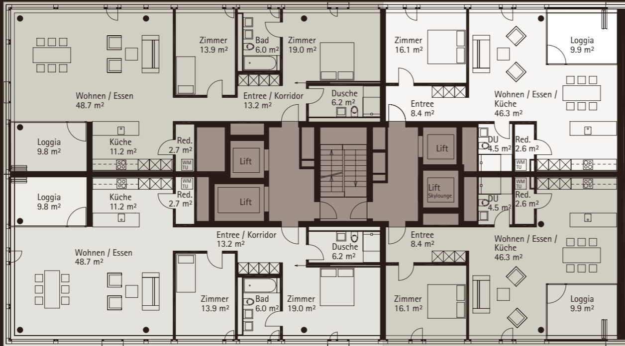
WOHNUNG 01.0902, 3 1/2-ZIMMER NGF: 121.0 m 2 , Loggia: 9.8 m 2
