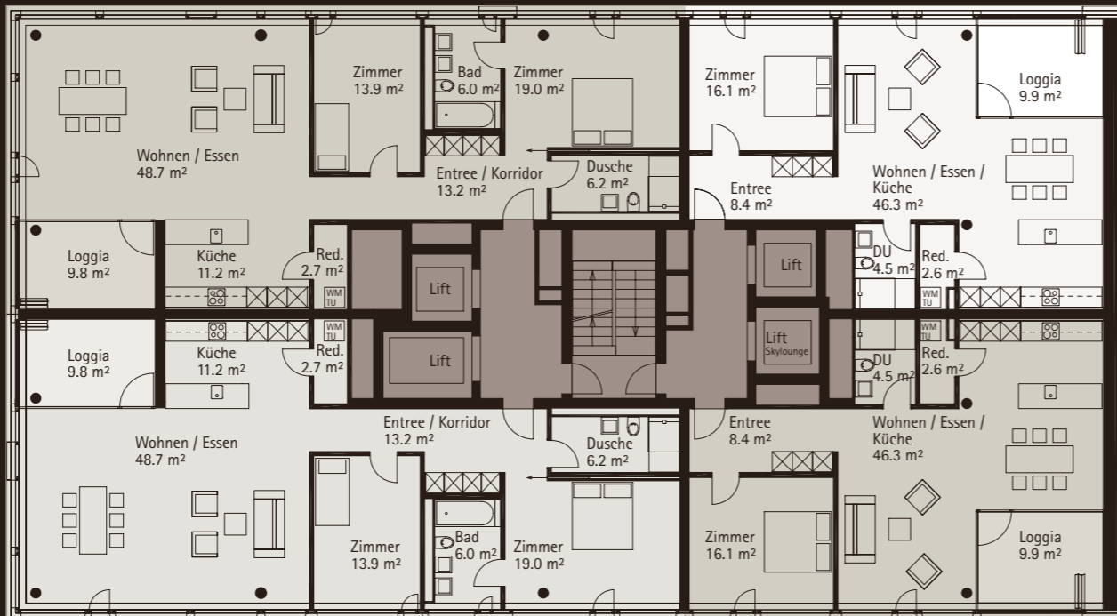
WOHNUNG 01.0802, 3½-ZIMMER NGF: 121.0 m 2 , Loggia: 9.8 m 2
