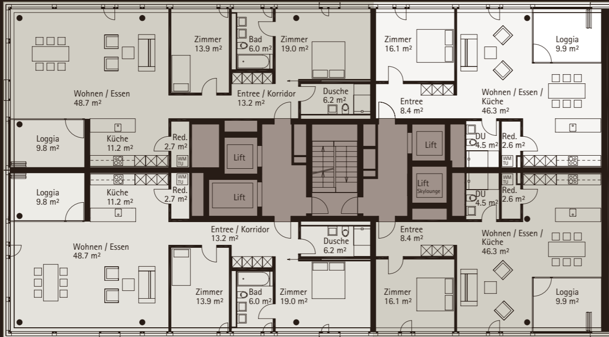
WOHNUNG 01.0902, 3½-ZIMMER NGF: 121.0 m 2 , Loggia: 9.8 m 2
